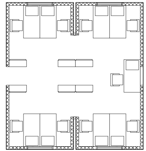
AVOIN TOIMISTO AUKKO 4m
