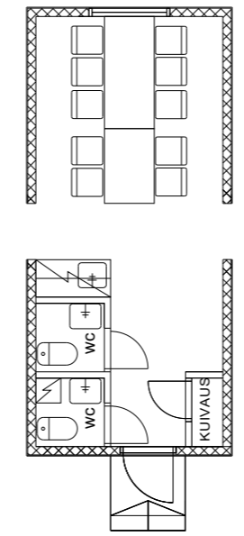
MINIKEITTIÖ / 2 X WC
