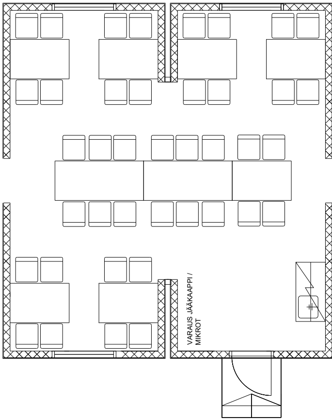
TAUKOTILA / MINIK. AUKKO 4m
